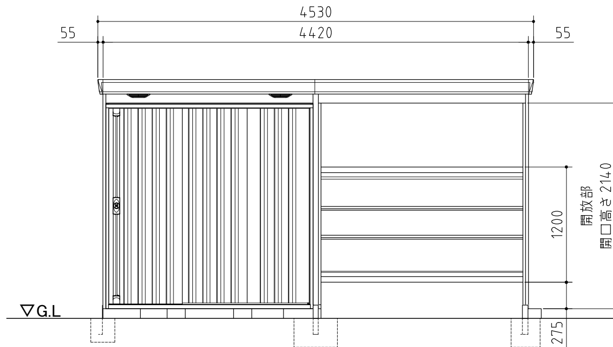
正面図
